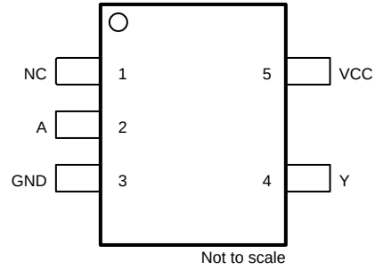
图 4-2. SN74LVC1G16-Q1 DCK 封装，5 引脚 SOT-SC70 (顶视图)
