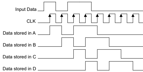
图 8-2. 应用时序图
