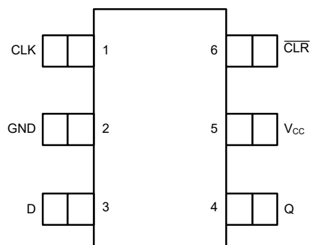
图 4-1. DBV 或 DCK 封装，6 引脚 SOT-23 或 SOT-SC70 (俯视图)
