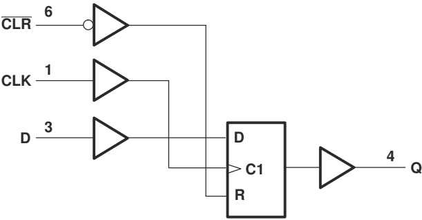
逻辑图
