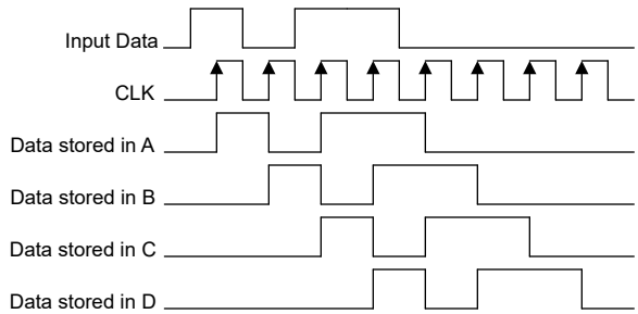
图 8-2. 应用时序图
