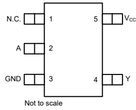
图 4-1. DCK、DBV 封装 5 引脚 SC70、SOT-23 顶视图
