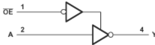
图 7-1. 逻辑图 (正逻辑)
