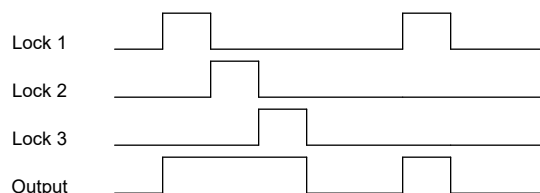
图 7-2. 互锁信号和逻辑输出
