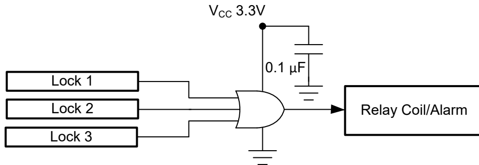
图 7-1. 典型应用图
