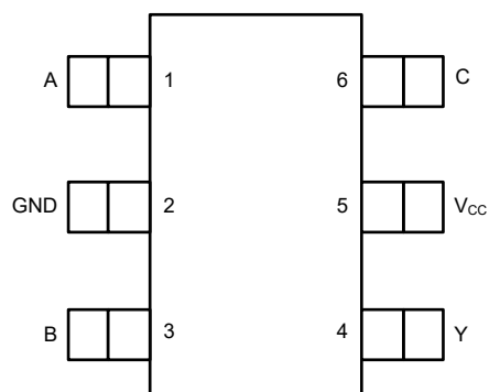
图 4-1. DBV 或 DCK 封装，6 引脚 SOT-23 或 SC-70 ( 顶视图 )
