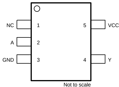
图 4-2. SN74LVC1G37 DCK 封装，5 引脚 SOT-SC70 (顶视图)
