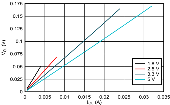
图 5-4. 低电平状态下输出电压与电流间的关系
