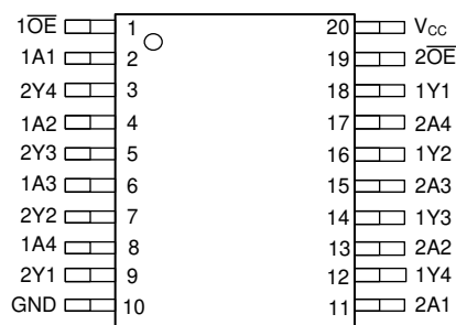
图 4-2. SN74LVC240A PW、DW、NS、DB、 DGS、DGV 封装 (顶视图)
