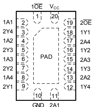
图 4-1. SN74LVC240A RKS 封装 (顶视图)
