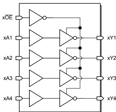
图 7-1. SN74LVC240A 的逻辑图 (正逻辑)
