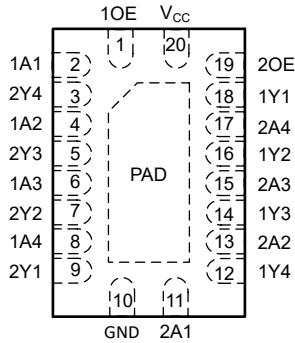
图 4-1. SN74LVC241A RKS 封装 (顶视图)
