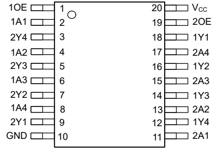
图 4-2. SN74LVC241A PW、DGS 封装 (顶视图)
