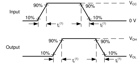
图 6-4. 电压波形，输入和输出转换时间
