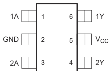
图 3-1. DBV 或 DCK 封装、6 引脚 SOT-23 或 SC70 ( 顶视图 )
