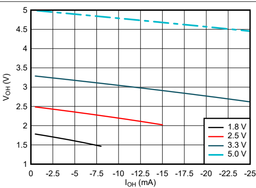
图 5-2. 高电平状态下输出电压与电流间的关系
