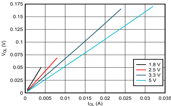
图 5-3. 低电平状态下输出电压与电流间的关系
