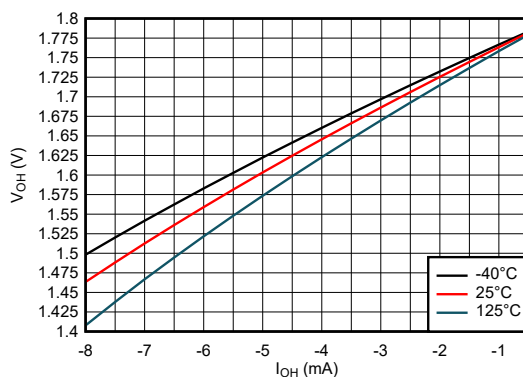
图 5-7. 高电平状态下输出电压与电流间的关系 (1.8V 电源)
