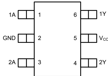
图 4-1. DBV , 6 引脚 SOT-23 ( 顶视图 )
