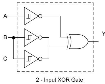
2 - Input XOR Gate
