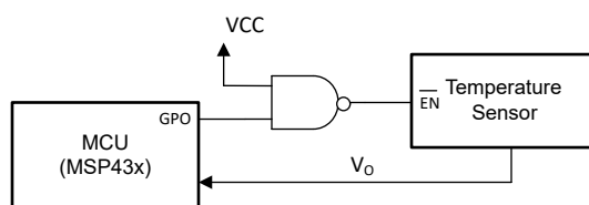
图 8-1. 典型应用原理图
