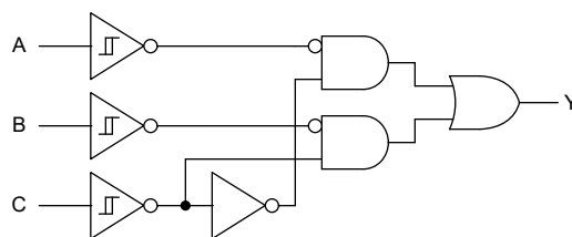
功能图
