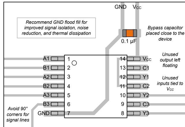
图 8-3. SN74LVC3G97-Q1 的示例布局
