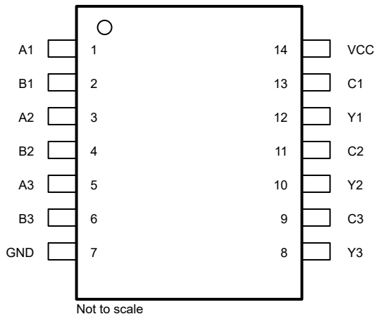
图 4-1. SN74LVC3G98-Q1 PW 封装 (预发布), 14 引脚 TSSOP (顶视图) 图 4-2. SN74LVC3G98-Q1 BQA 封装, 14 引脚 WQFN (顶视图)
