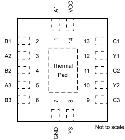
图 4-1. SN74LVC3G98-Q1 PW 封装 (预发布), 14 引脚 TSSOP (顶视图) 图 4-2. SN74LVC3G98-Q1 BQA 封装, 14 引脚 WQFN (顶视图)
