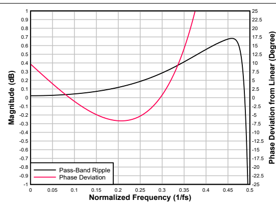
图 6-51. 超低延迟抽取滤波器通带纹波和相位偏差
