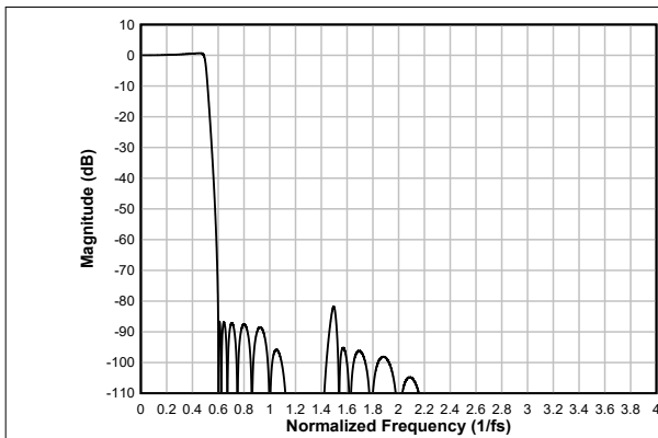
图 6-50. 超低延迟抽取滤波器幅度响应
