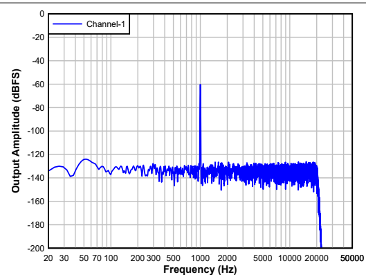
图 8-3. 具有-60dBFS 输入的 ADC FFT
