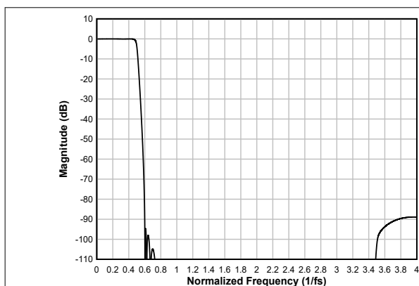
图 6-77. 低延迟内插滤波器幅度响应
