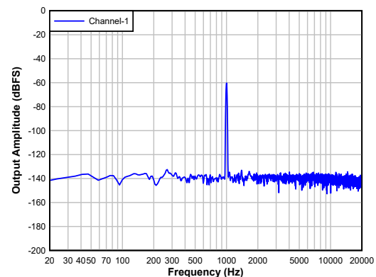
图 8-5. 具有-60dBFS 输入的 DAC FFT
