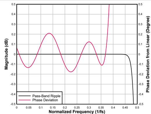
图 6-86. 低延迟内插滤波器通带纹波和相位偏差
