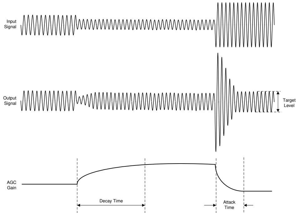
图 6-60. AGC 特性
