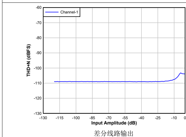
图 8-4. DAC THD+N 级别与输入间的关系
