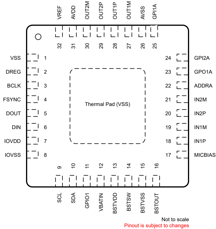
图 4-2. TAC5312-Q1 RTV 封装, 32 引脚 WQFN (带有外露散热焊盘), 顶视图
