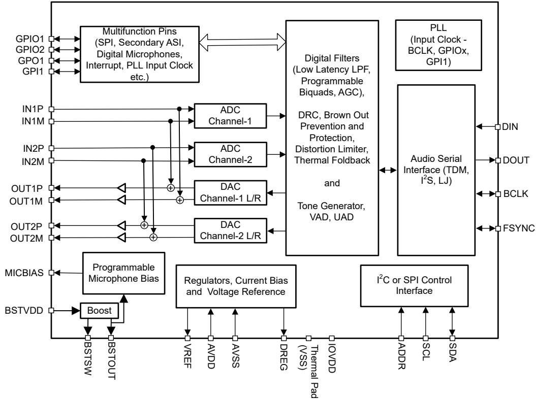
图 6-1. 功能方框图
