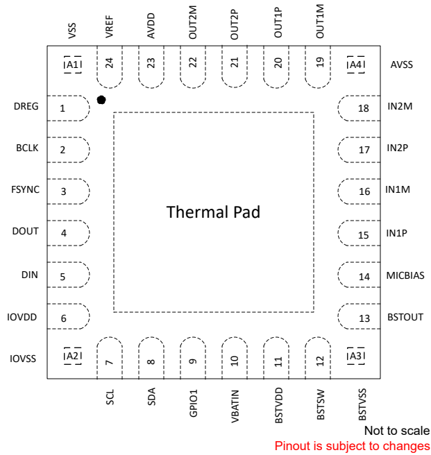
图 4-1. TAC5312-Q1 RGE 封装，28 引脚 WQFN (带有外露散热焊盘)，顶视图
