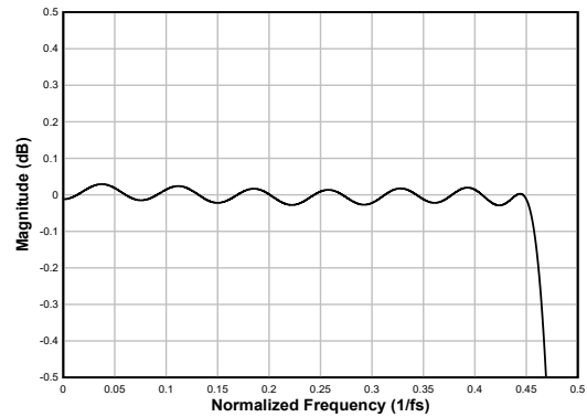
图 6-41. 线性相位内插滤波器通带纹波
