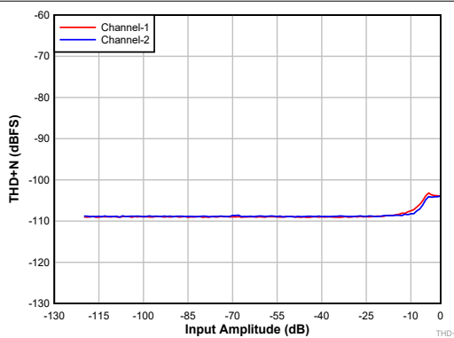
图 7-2. DAC THD + N 级别与输入间的关系
