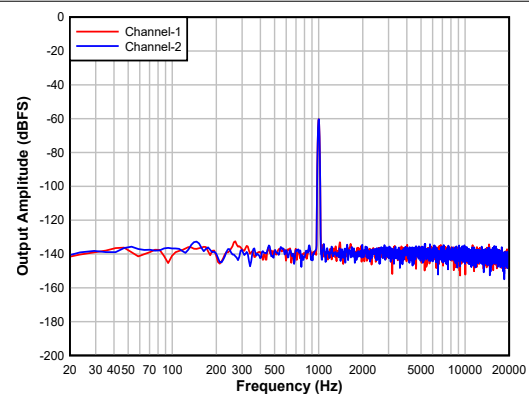
图 7-3. DAC FFT
