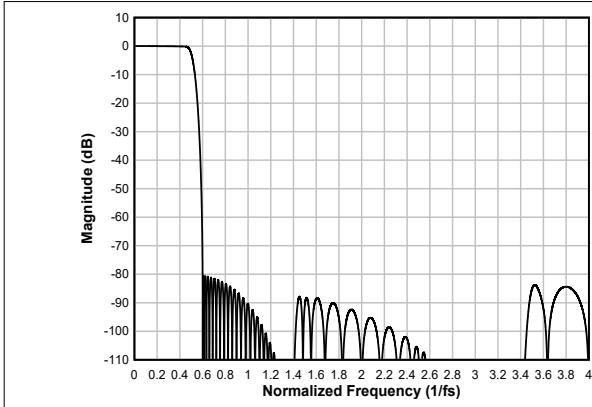
图 6-24. 线性相位内插滤波器幅度响应
