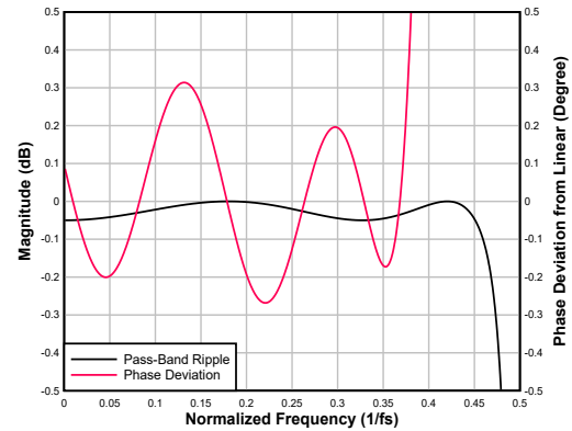
图 6-47. 低延迟内插滤波器通带纹波和相位偏差
