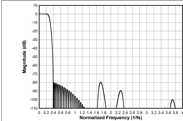
图 6-76. 线性相位抽取滤波器幅度响应
