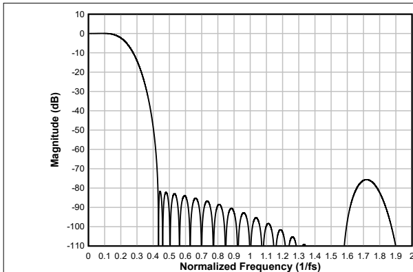
图 6-78. 线性相位抽取滤波器幅度响应
