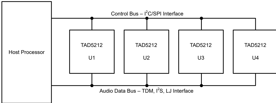
图 7-14. 多个 TAD5212 器件具有共享控制和音频数据总线
