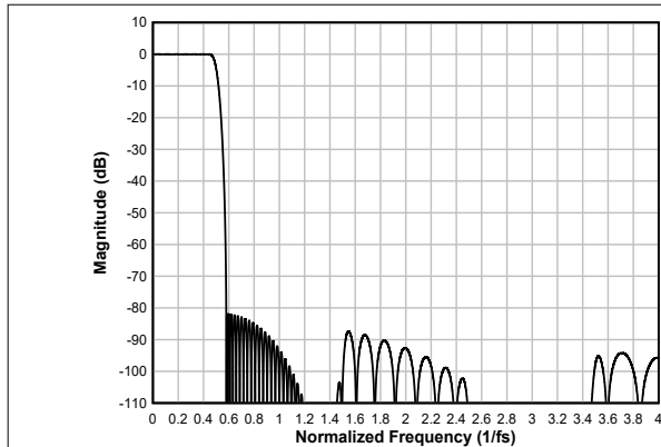
图 6-28. 线性相位内插滤波器幅度响应
