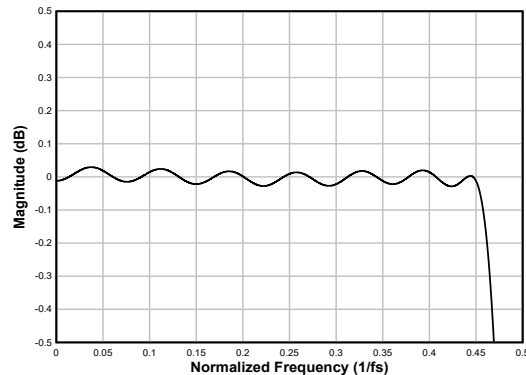
图 7-22. 线性相位内插滤波器通带纹波
