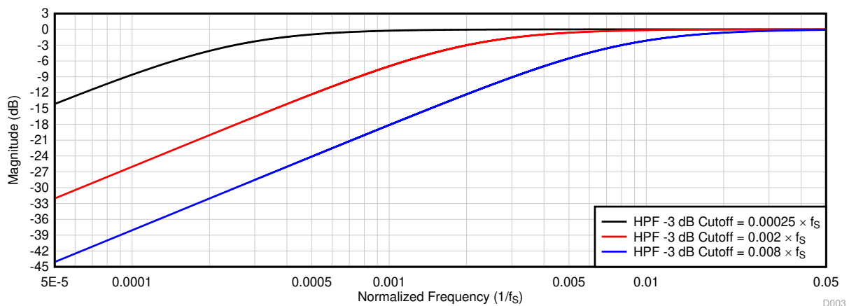
图 6-61. HPF 滤波器频率响应图
