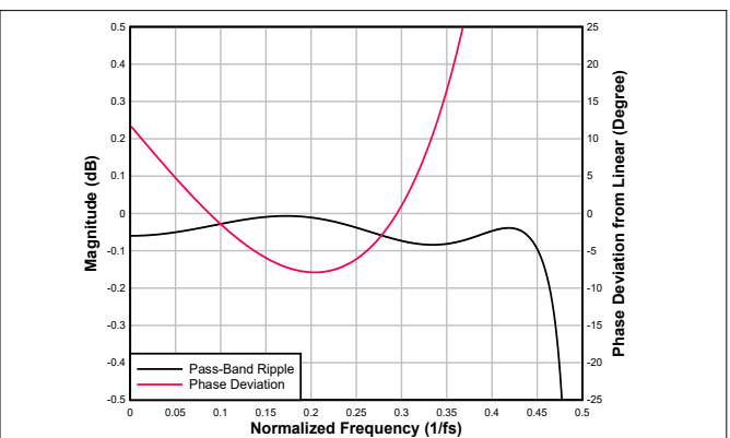
图 6-55. 超低延迟内插滤波器通带纹波和相位偏差
