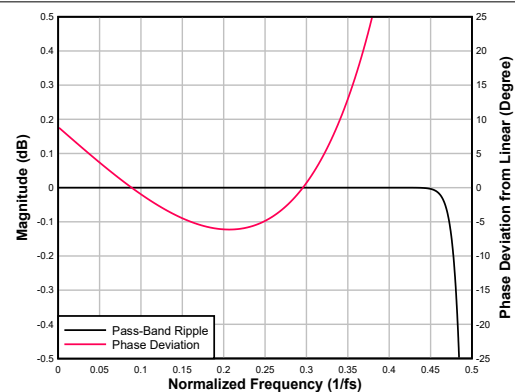
图 6-59. 超低延迟内插滤波器通带纹波和相位偏差
