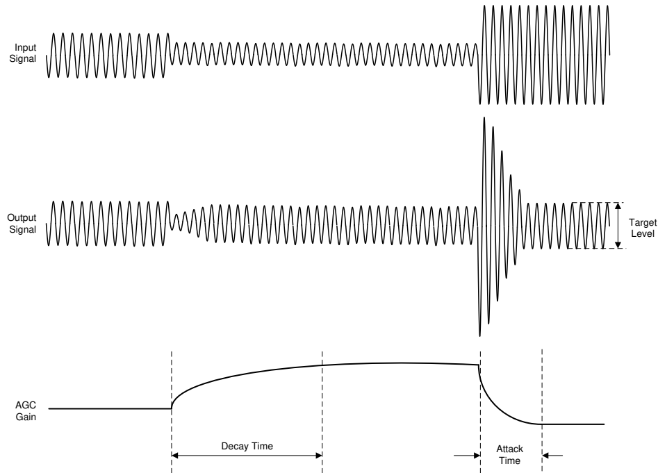
图 6-100. AGC 特性
