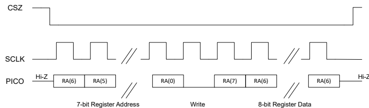
图 6-106. SPI 单字节写入传输
