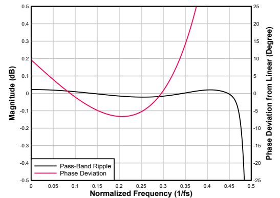
图 6-95. 超低延迟抽取滤波器通带纹波和相位偏差
