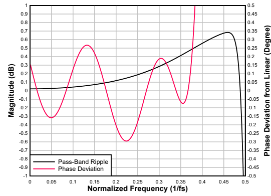
图 6-83. 低延迟抽取滤波器通带纹波和相位偏差
