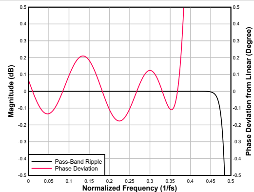
图 6-49. 低延迟内插滤波器通带纹波和相位偏差
