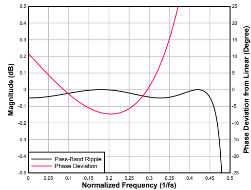
图 6-57. 超低延迟内插滤波器通带纹波和相位偏差
