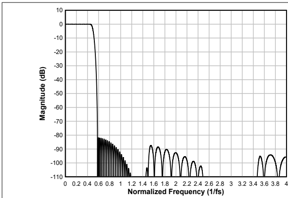
图 6-26. 线性相位内插滤波器幅度响应
