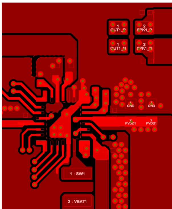
图 8-4. 示例布局顶部
