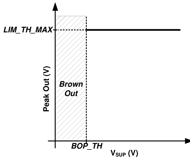
图 6-4. 具有固定阈值的限制器
