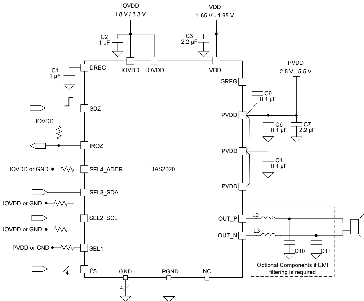
图 8-1. 外部 PVDD 系统的应用示意图
