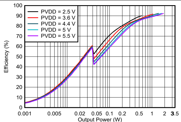
图 8-3. 效率与输出功率间的关系
