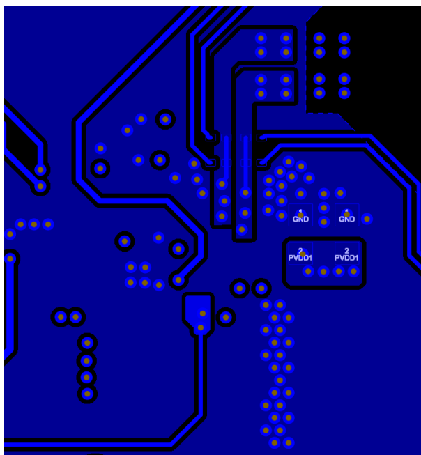
图 8-5. 示例布局底部
