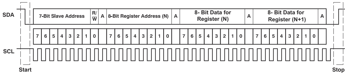
图 6-7. 典型的 I 2 C 序列
