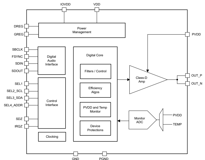
功能方框图
