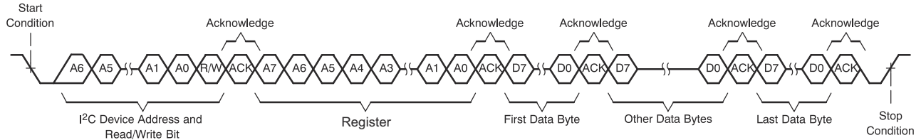
图 6-9. I 2 C 多字节写入传输
