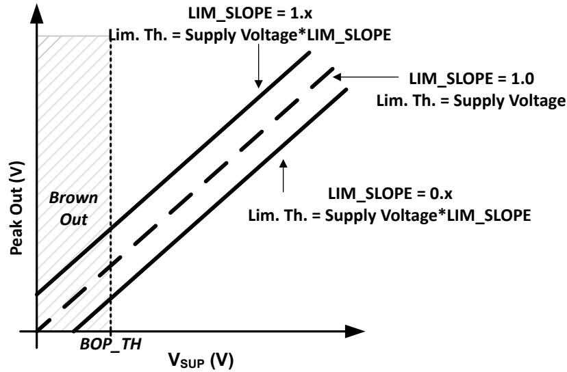
图 6-3. 具有动态电源余量的限制器
