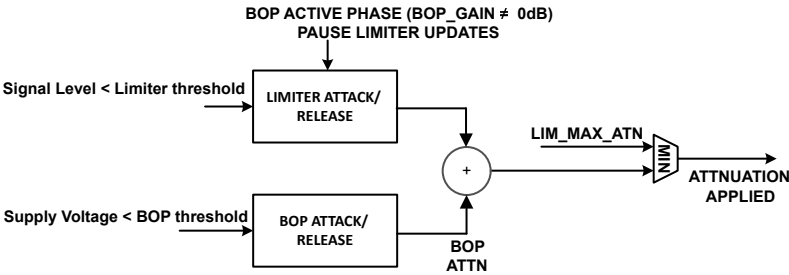
图 6-2. 限制器和欠压增益衰减
