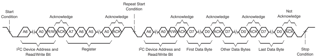
图 6-11. I 2 C 多字节读取传输
