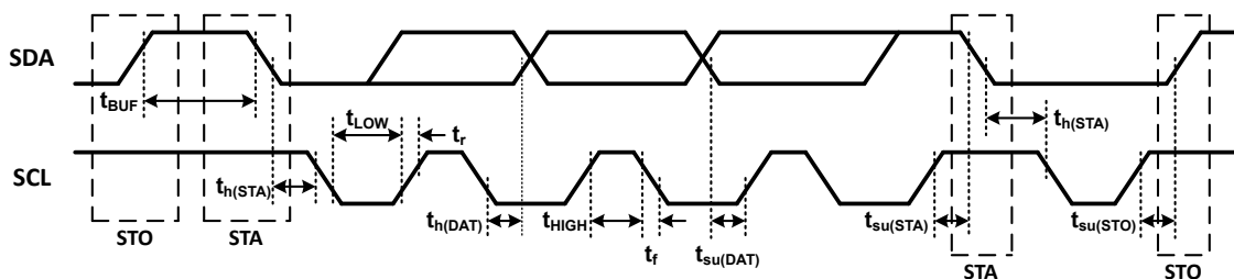
图 5-1. I 2 C 时序图
