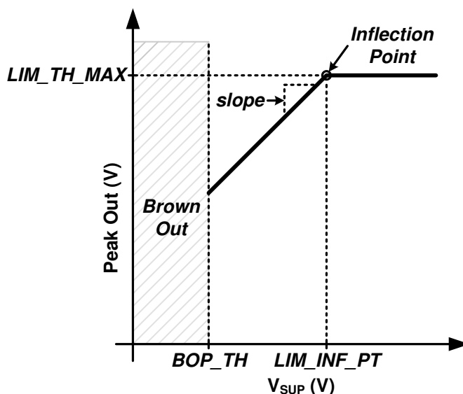
图 6-5. 具有拐点的限制器
