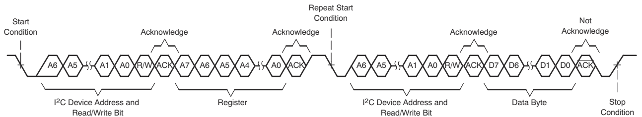
图 6-10. I 2 C 单字节读取传输
