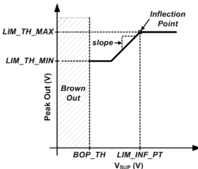
图 6-6. 具有拐点和最小阈值的限制器
