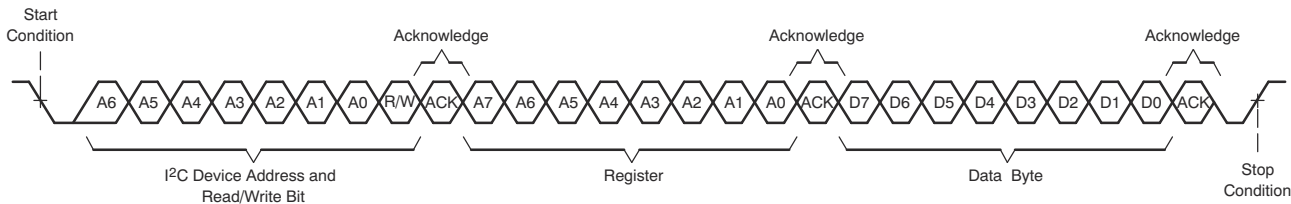
图 6-8. I 2 C 单字节写入传输
