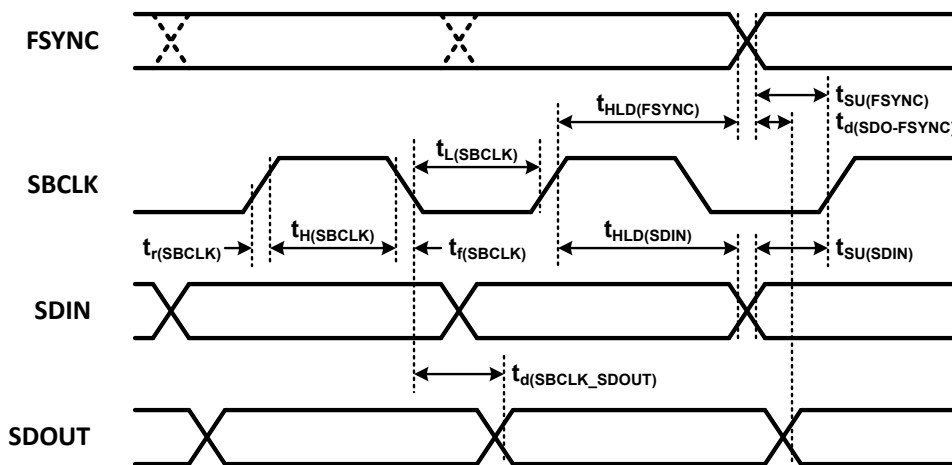
图 5-2. I 2 S/TDM 时序图
