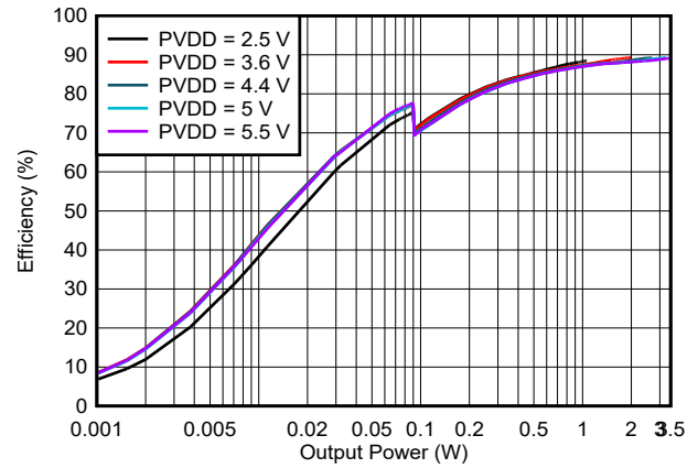
图 5-10. 效率与输出功率间的关系
