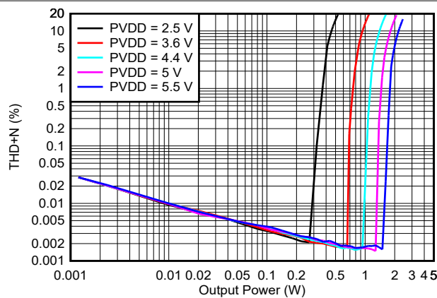
图 8-2. THDN 与输出功率间的关系
