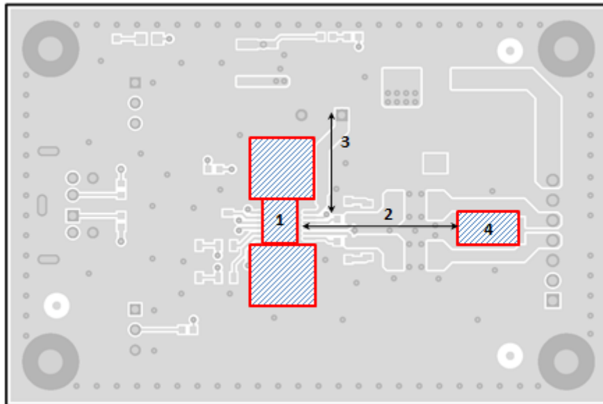
Figure 18. Top Layer
