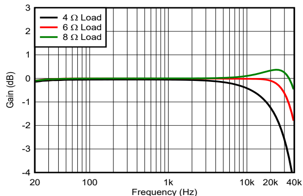
图 5-60. 增益与频率间的关系
