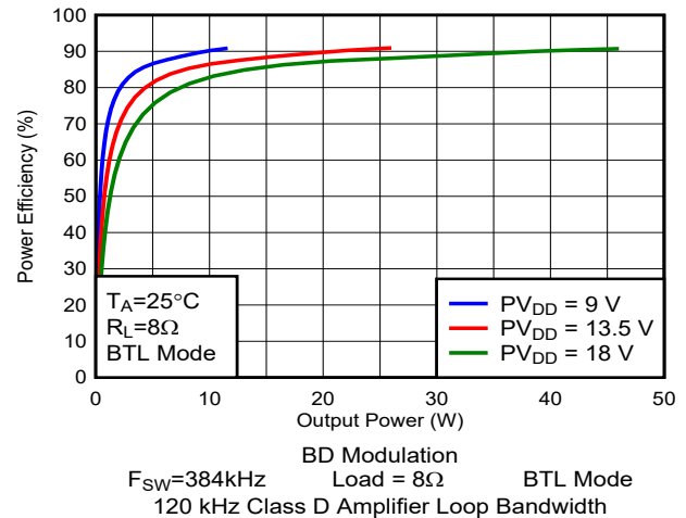
图 5-66. 效率与输出功率间的关系
