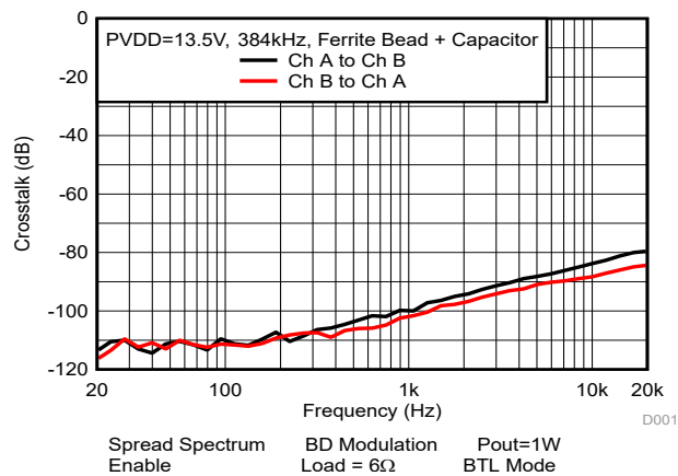
图 5-63. 串扰
