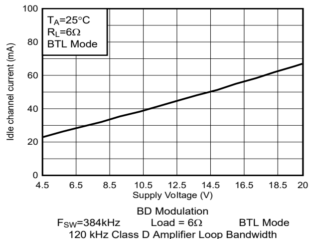
图 5-64. PVDD 空闲电流与 PVDD 电压间的关系
