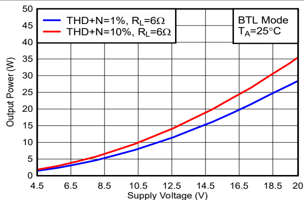
图 5-19. 输出功率与电源电压间的关系
