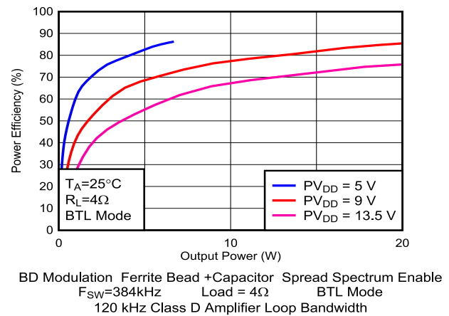
图 5-68. 效率与输出功率间的关系 (带 FB)
