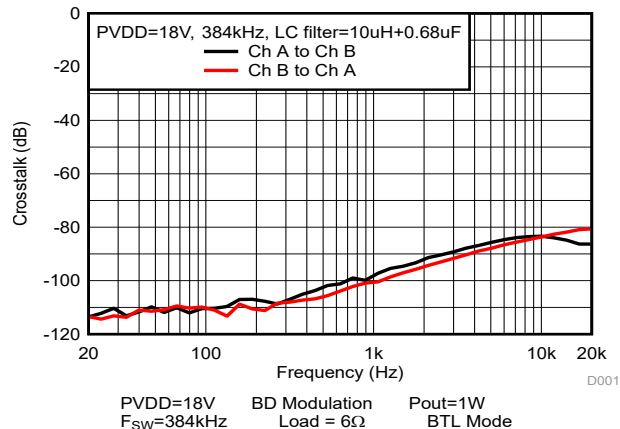
图 5-62. 串扰
