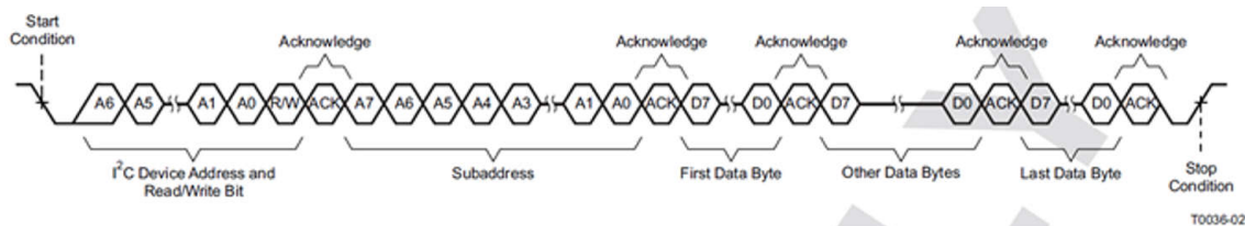
图 6-13. 顺序写入传输
