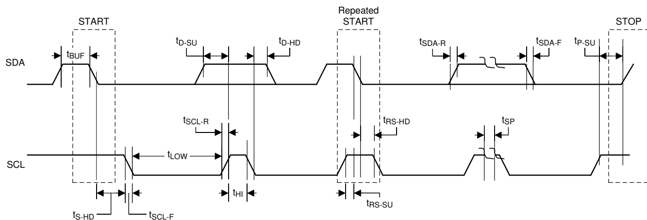
图 6-8. I²C 通信时序 - 目标
