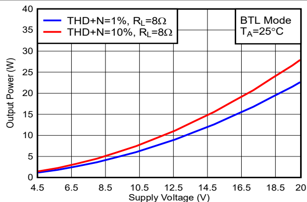
图 5-20. 输出功率与电源电压间的关系
