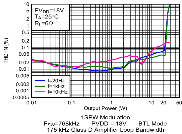
图 5-15. THD+N 与输出功率间的关系
