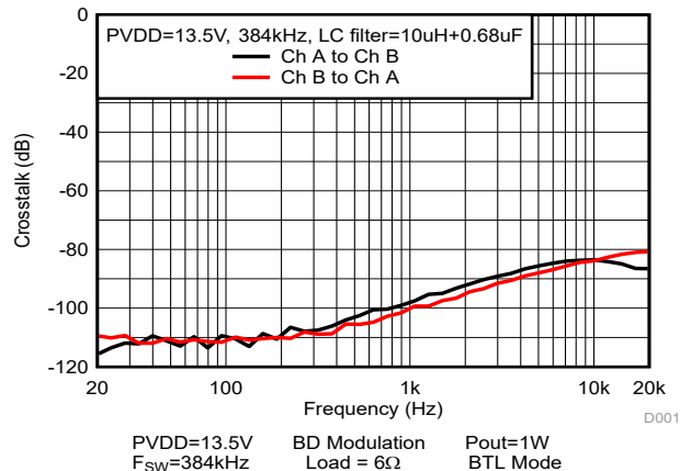
图 5-61. 串扰
