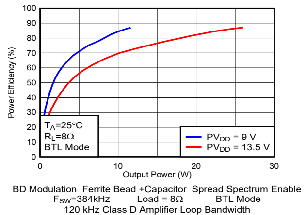
图 5-70. 效率与输出功率间的关系
