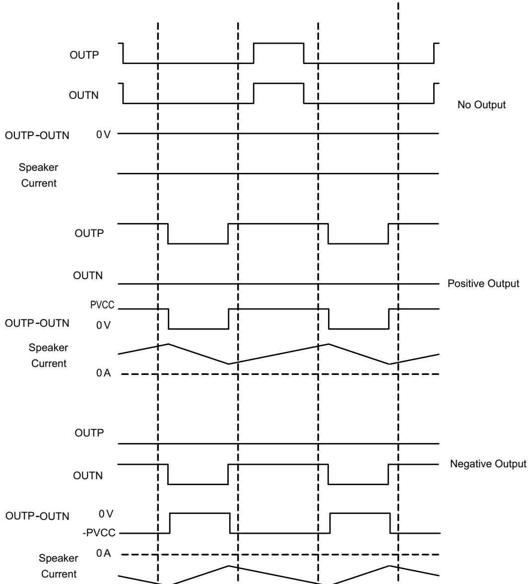
图 6-11. 1SPW 模式调制
