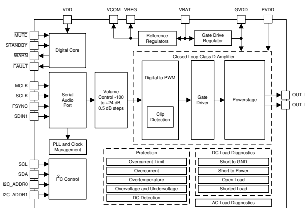
功能方框图
