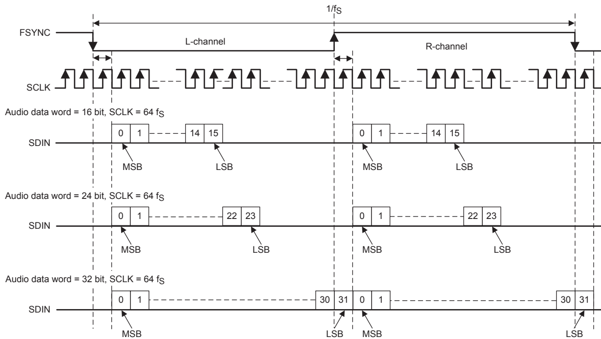
图 27. I 2 S Audio Data Format
