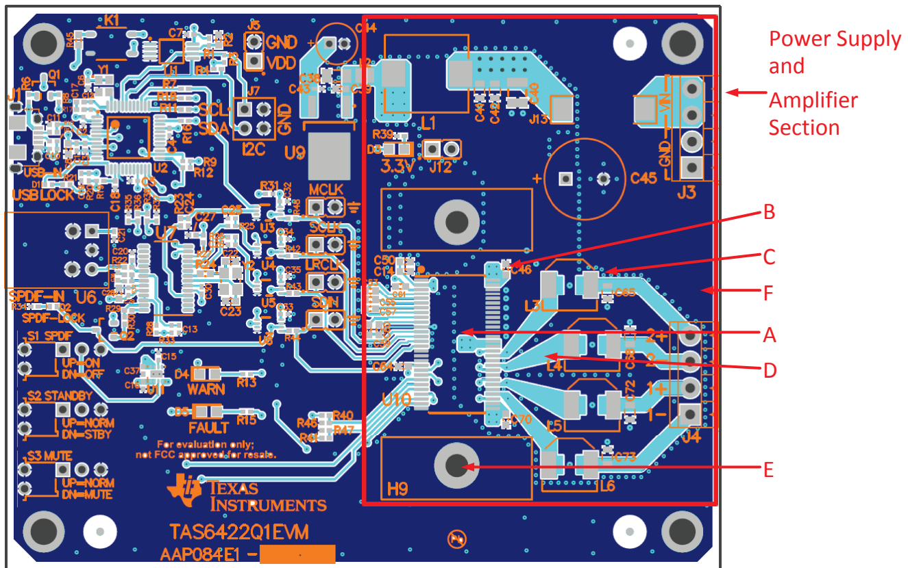
图 79. EVM Layout
