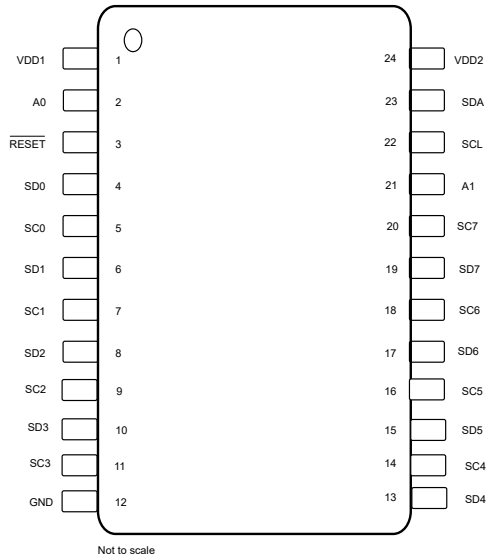
图 4-1. PW 封装，24 引脚 TSSOP ( 俯视图 )
