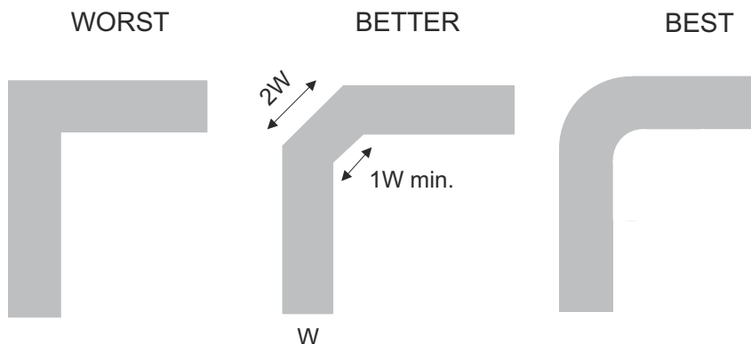
图 8-7. 布局原理图
