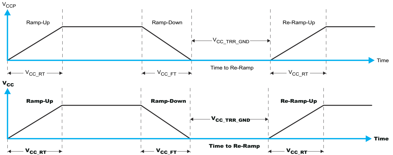
图 8-6. 将 V_{CCP} 降至 0.2V 或 0V 以下，然后上升
