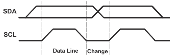
图 7-5. 位传输
