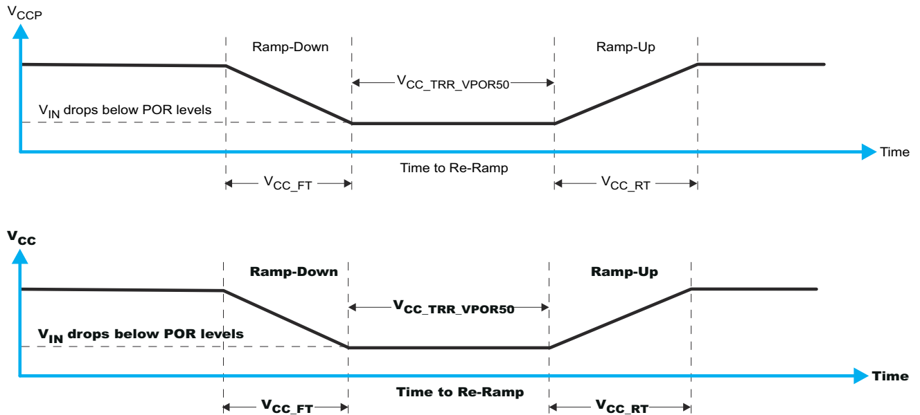
图 8-7. 将 V_{CCP} 降至低于 POR 阈值，然后重新上升
