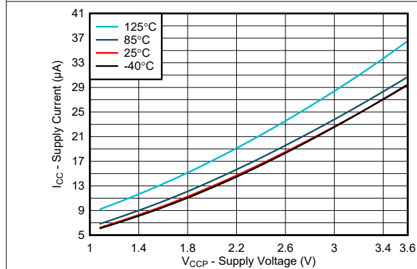
图 5-5. 电源电流与电源电压的关系 - FM+ 模式
