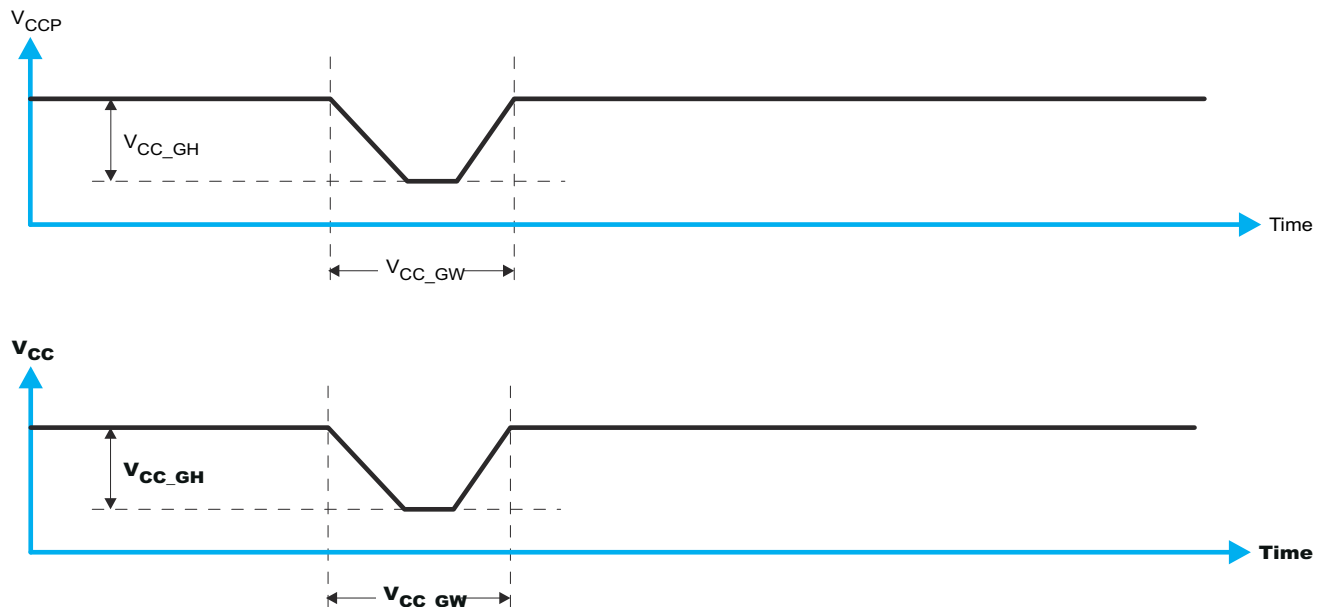
图 8-8. 干扰宽度和干扰高度
