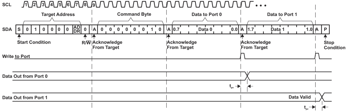
图 7-9. 对输出端口寄存器进行写入
