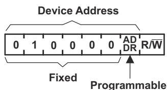
图 7-7. TCAL6408 地址
