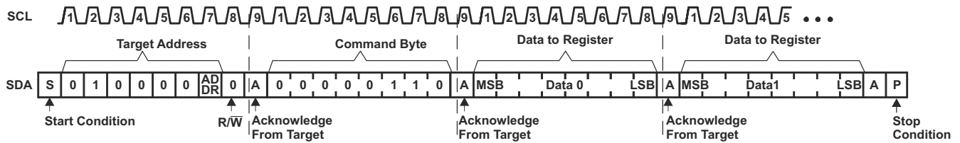
图 7-10. 写入配置寄存器或极性反转寄存器
