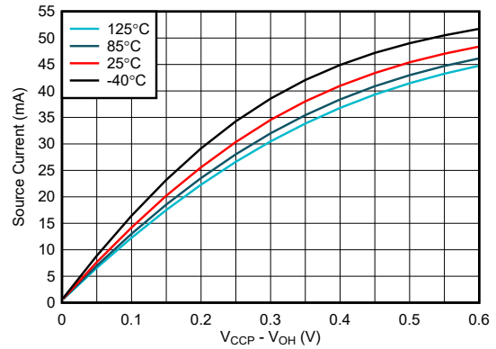
图 5-14. I/O 拉电流与输出高电压的关系， V CCP = 1.2V
