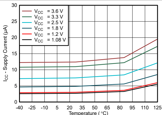
图 6-1. 电源电流与温度间的关系 - FM 模式
