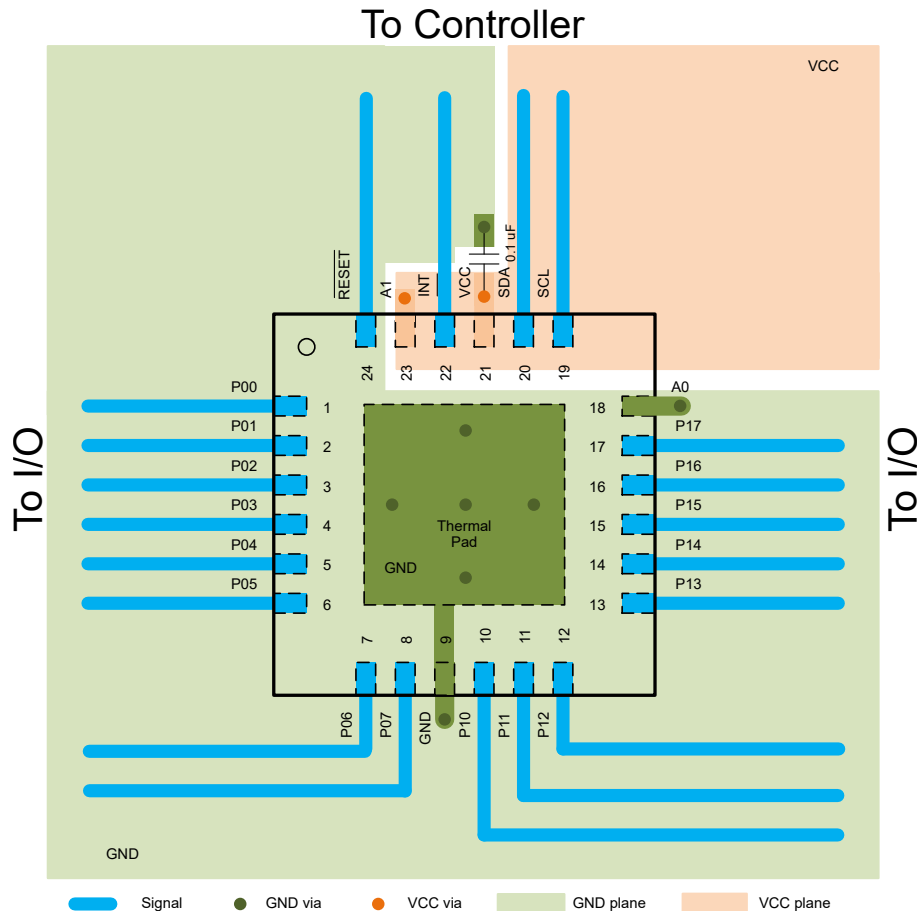
图 9-10. TCAL9539-Q1 布局
