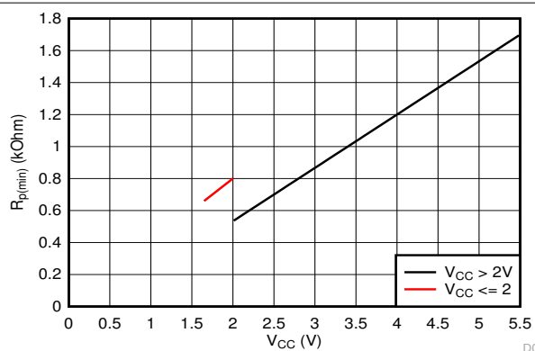
图 9-5. 最小上拉电阻 ( R_{p(min)} ) 与上拉基准电压 ( V_{CC} ) 间的关系
