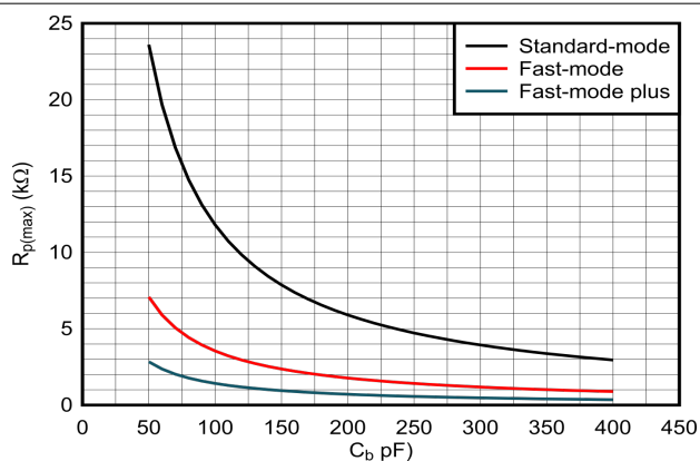
图 9-4. 最大上拉电阻 ( R_{p(max)} ) 与总线电容 ( C_b ) 间的关系
