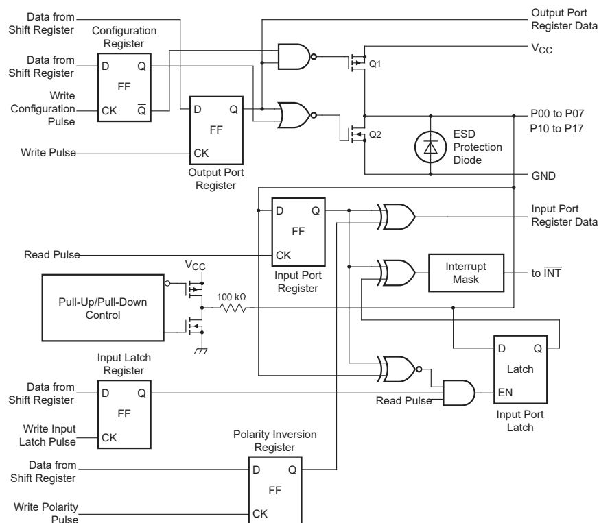
图 8-2. P00 至 P17 的简化原理图
