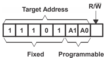
图 8-7. TCAL9539-Q1 地址
