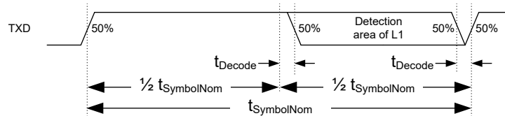
图 7-11. FAST TX 模式下 TXD 上的 Level_1 检测
