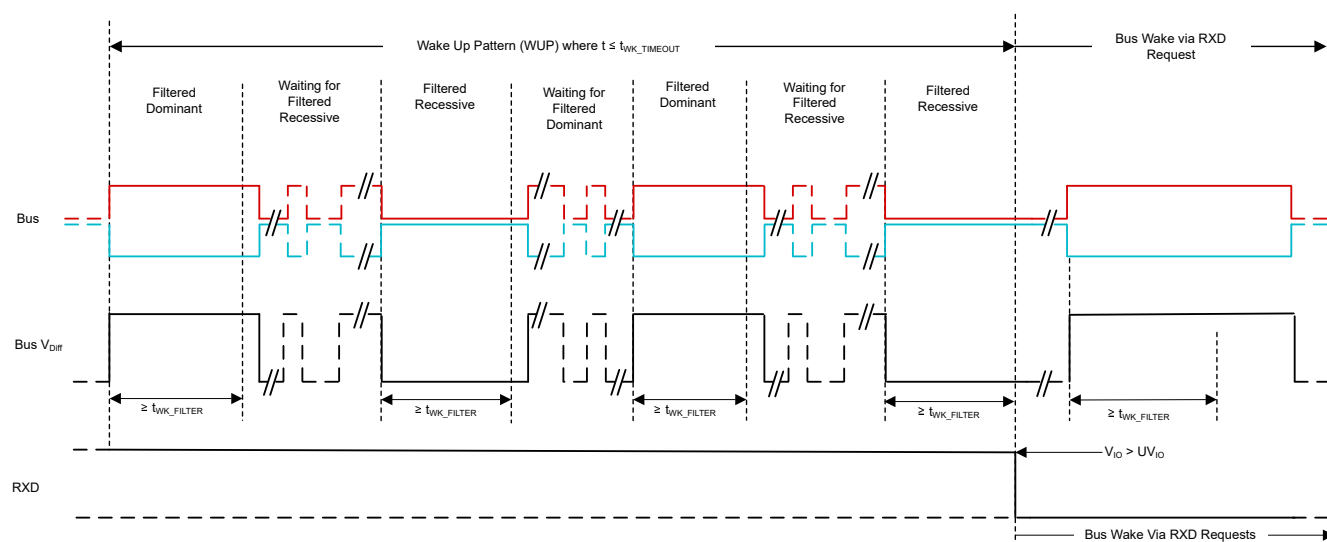
图 7-14. 具有 t_{WK\_TIMEOUT} 的唤醒模式 (WUP)
