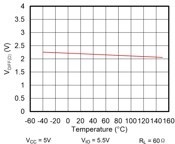
图 5-2. V_{DIFF(D)} 与温度间的关系
