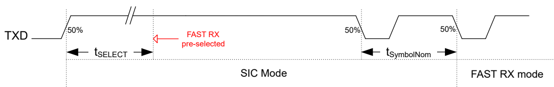
图 7-7. FAST RX 模式选择
