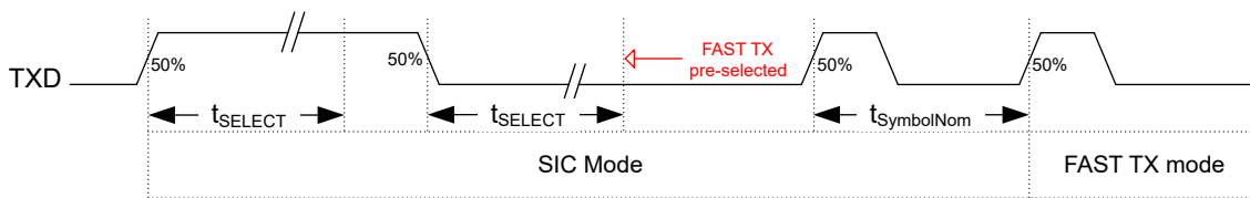
图 7-8. FAST TX 模式选择
