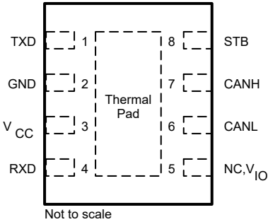
图 4-2. VSON (DRB) 封装，8 引脚 ( 顶视图 )
