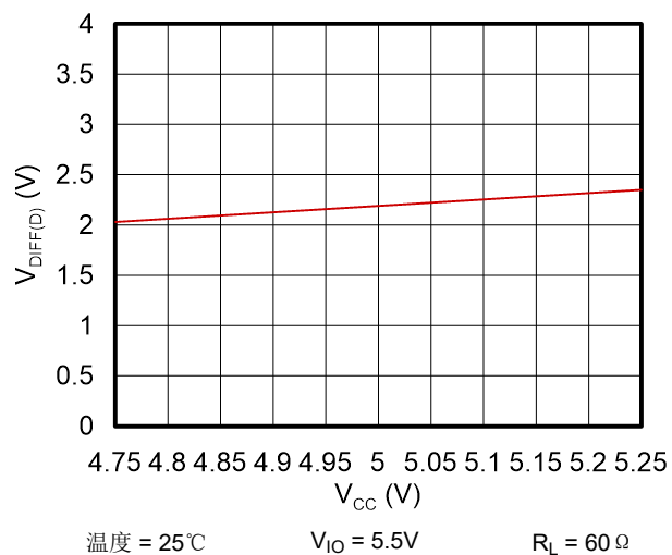
图 5-3. V_{DIFF(D)} 与 V_{CC} 间的关系
