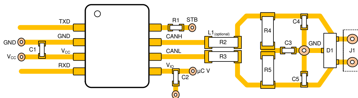
图 8-6. 布局示例
