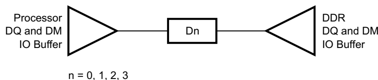
图 7-79. DQ/DM Topology
