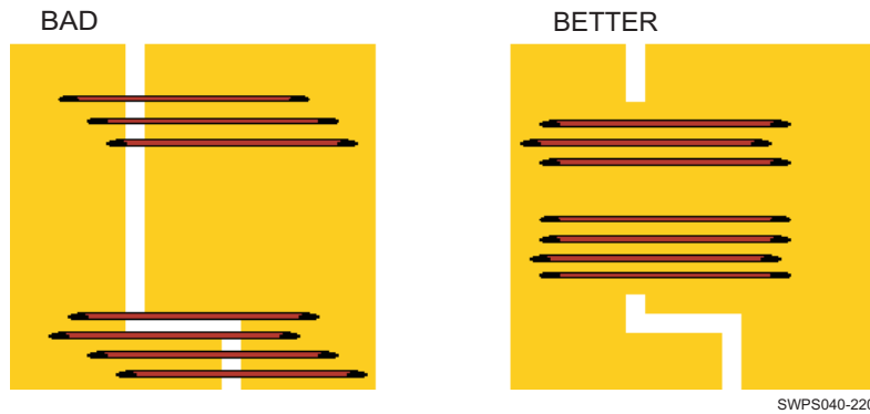
图 7-17. Trace Examples
