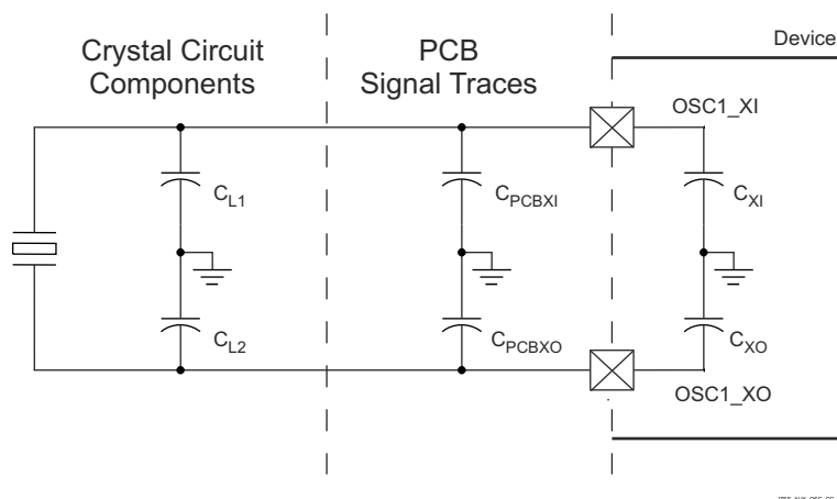
图 6-32. 负载电容
