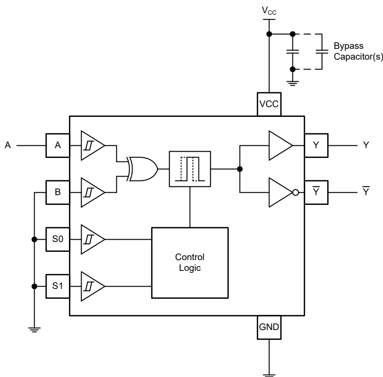
图 8-1. 使用 TDEL1G522 的延迟原理图
