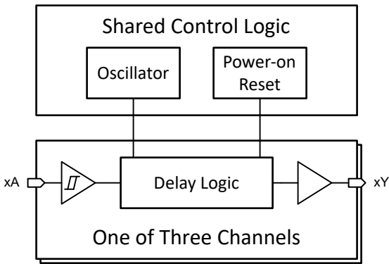
功能方框图
