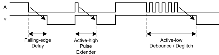
图 8-2. 输出时序图
