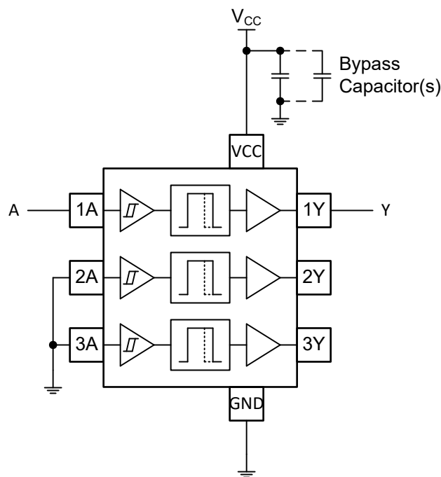
图 8-1. 使用 TDEL3G510-Q1 的下降沿延迟原理图
