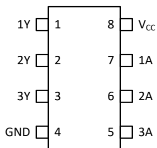
图 4-1. TDEL3G510-Q1 DRL 封装 ( 顶视图 )
