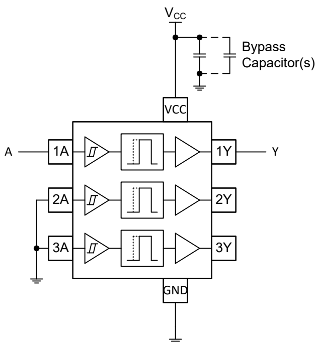
图 8-1. 使用 TDEL3G511 的上升沿延迟原理图
