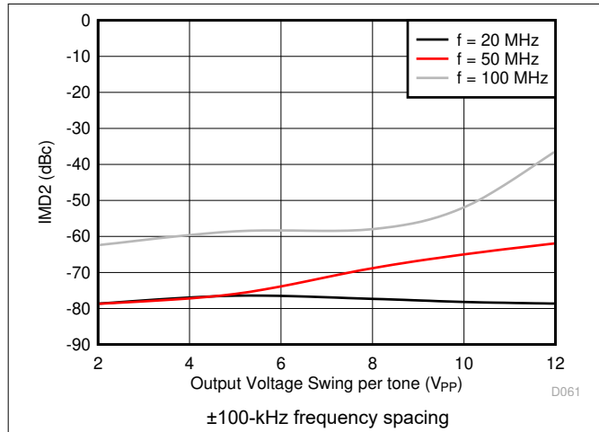
图 8-19. IMD2 vs Output Voltage Swing
