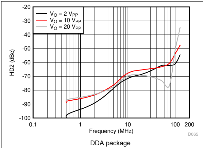
图 8-7. HD2 vs Frequency
