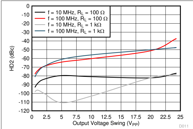
图 8-13. HD2 vs Output Swing
