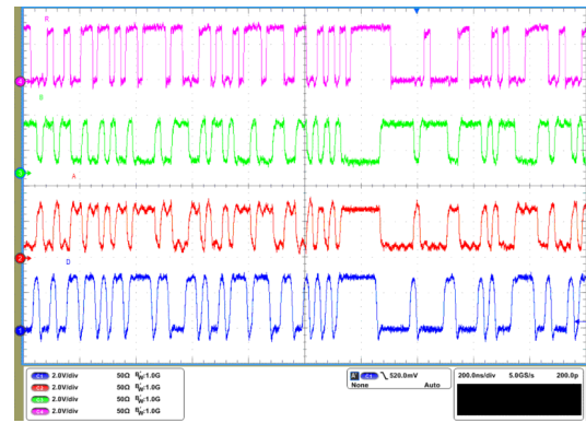
THVD2450V-EP V_{CC} = 3.3V R_L = 50\Omega 50Mbps 下的随机 (PRBS7) 数据
