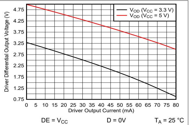
图 5-2. 驱动器差分输出电压与驱动器输出电流的关系
