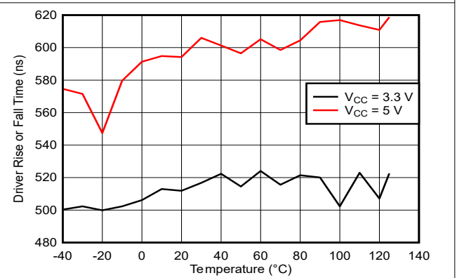
图 5-4. THVD2410V-EP 驱动器上升时间或下降时间与温度之间的关系
