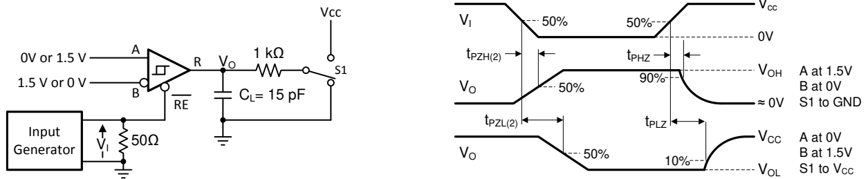
图 6-7. 驱动器已启用情况下接收器启用/禁用次数的测量
