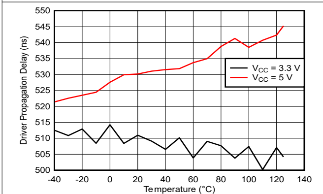
图 5-5. THVD2410V-EP 驱动器传播延迟与温度之间的关系
