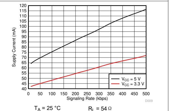
图 5-6. THVD2410V-EP 电源电流与信号速率间的关系
