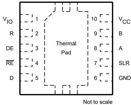
图 4-1. THVD2410V-EP、THVD2450V-EP 10 引脚 DRC 封装 (VSON) (顶视图)
