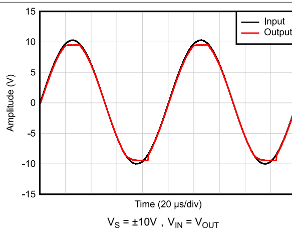
图 5-26. 无相位反转
