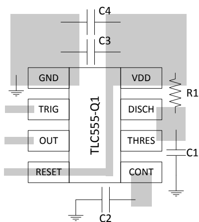
图 7-9. 建议布局
