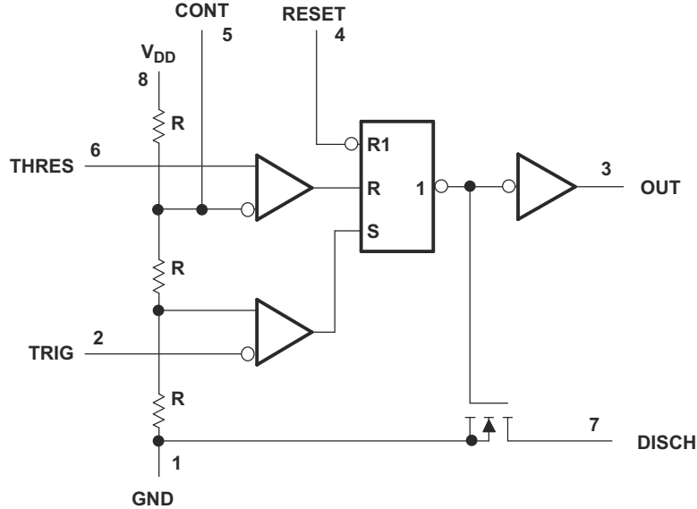
图 6-1. 简化原理图
