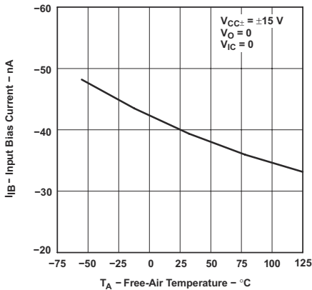
图 5-7. TLE2021xM 输入偏置电流与自然通风温度间的关系
