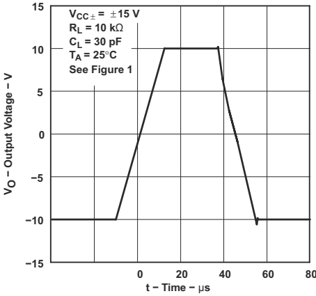
图 5-49. TLE2022xM 电压输出器大信号脉冲响应
