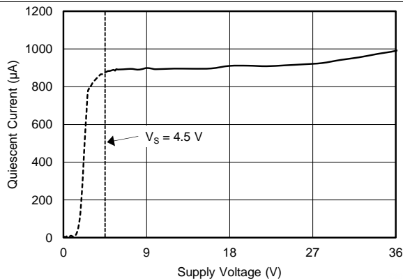
图 17. 静态电流与电源电压间的关系
