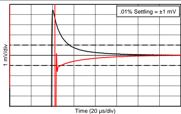
10V 正阶跃
