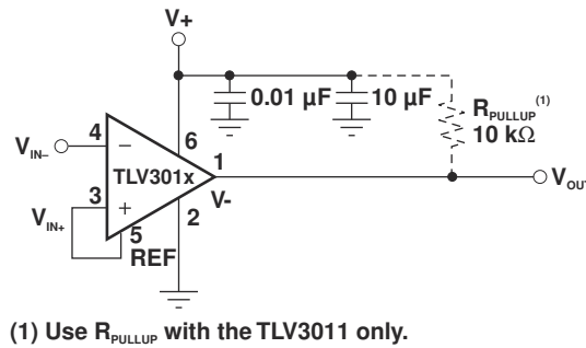
图 10-1. 基本连接
