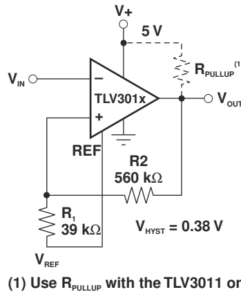
图 10-2. 添加迟滞
