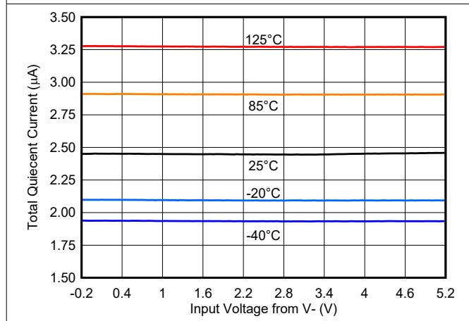
图 8-11. 电源电流与共模间的关系 - 5V
