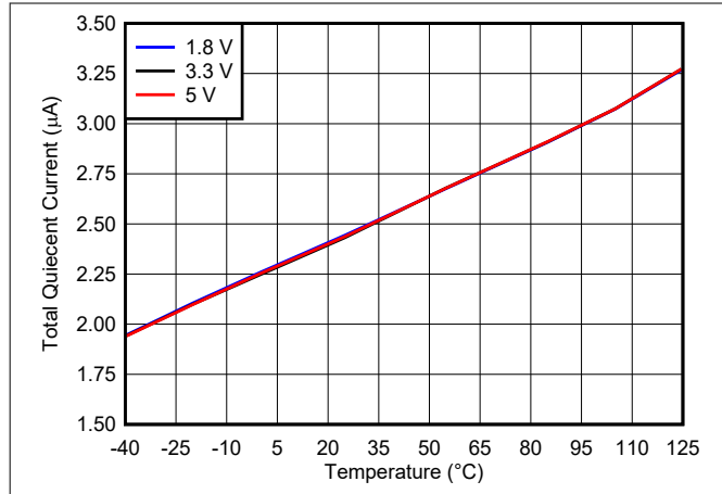
图 8-7. 电源电流与温度间的关系
