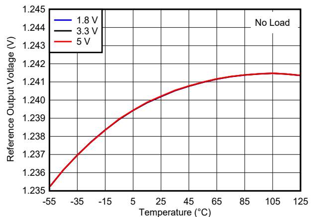
TLV3012-EP 基准电压与温度间的关系
