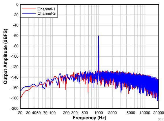
图 7-14. FFT With a -60-dBr Input
