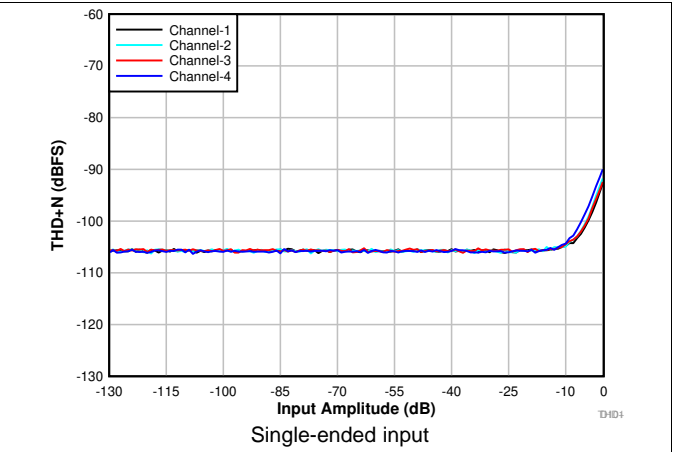
图 6. THD+N vs Input Amplitude
