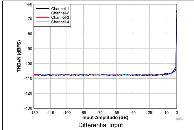
图 5. THD+N vs Input Amplitude
