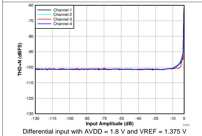
图 7. THD+N vs Input Amplitude
