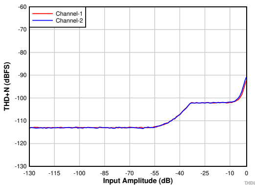
图 7-6. THD+N vs Input Amplitude With DRE Enabled
