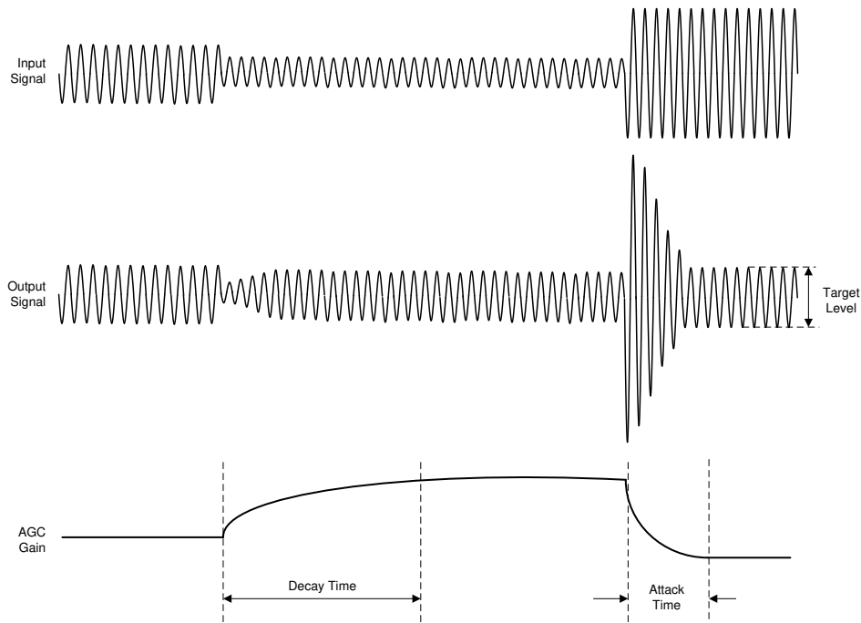
图 8-63. AGC Characteristics
