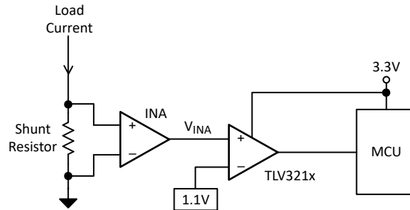
图 7-7. 电流检测
